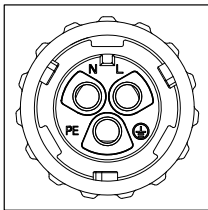
图4.15 交流电网终端连接器内部结构
