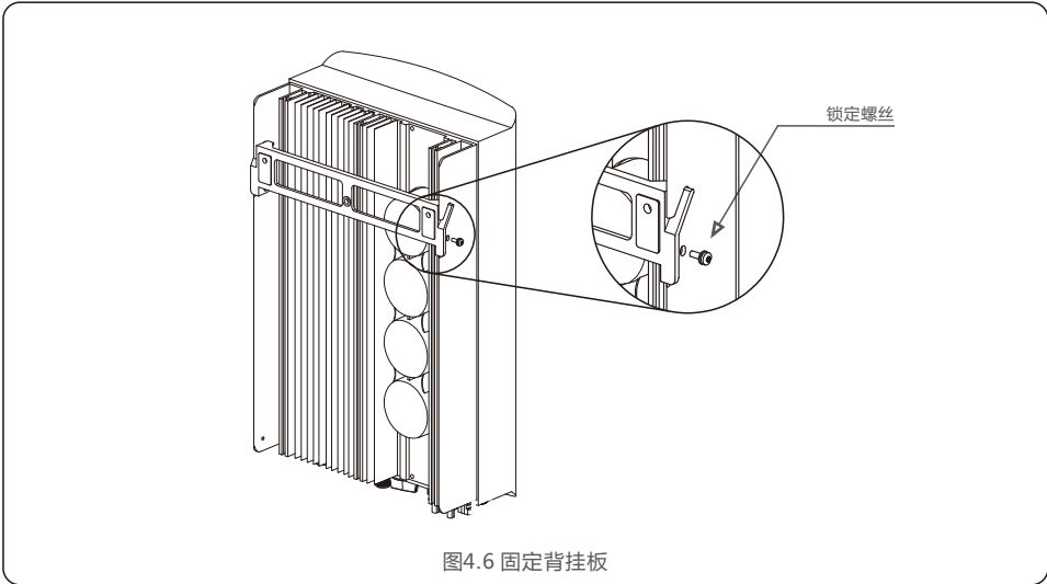
图4.6 固定背挂板 5. 使用配件中的螺钉，从逆变器底部将逆变器固定在背挂板上。（如图4.6）。
