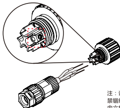
图 4.18 连接电缆线
