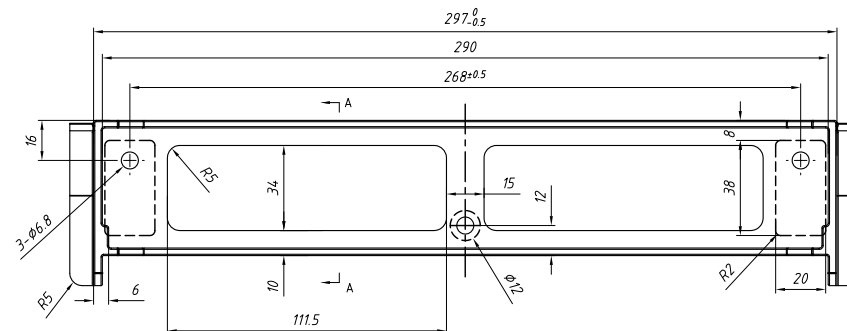
图4.3 逆变器安装
